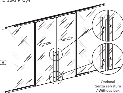
Porta scorrevole doppia anta in vetro /Double sliding glass door
